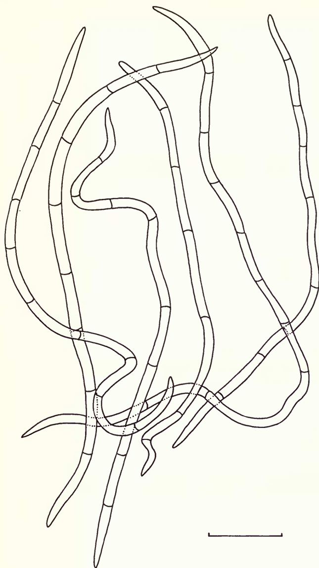
Fig. 36 Ascospore outlines of Celothelium dominicanum (Vainio) Aguirre (TUR 32697-holotype); scale = 10 \mu m.
